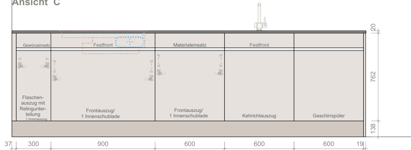
Ansicht C
