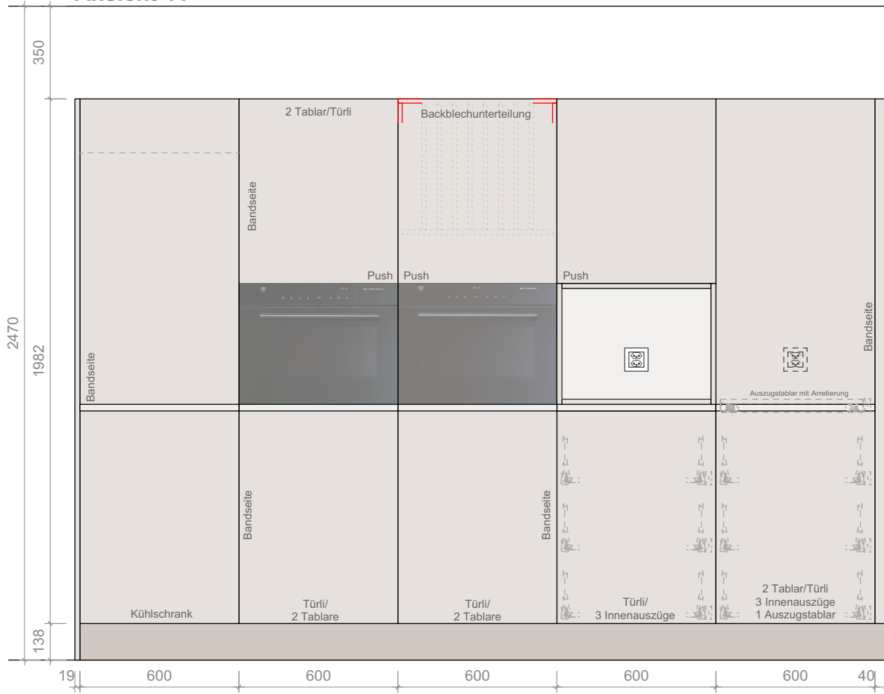
Ansicht A
