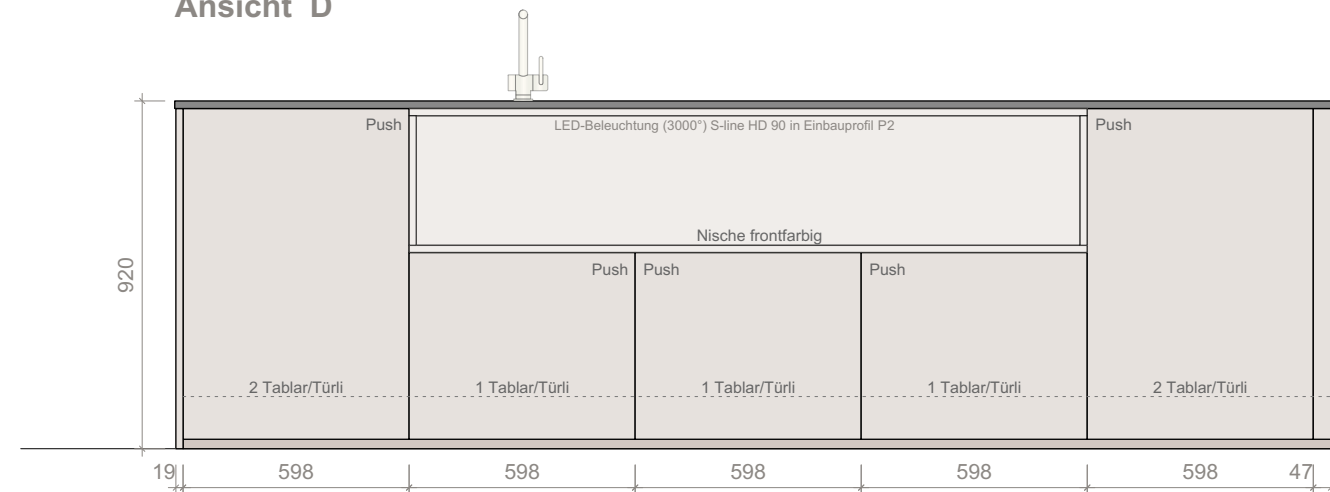
Ansicht D
